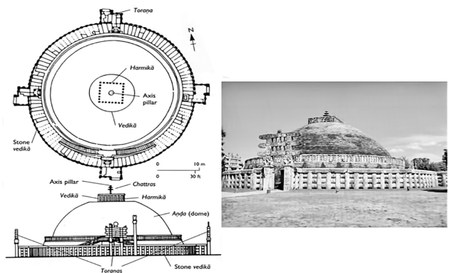
Hình 1. Bố cục Stupa ở Sanchi, Ấn Độ [1]
